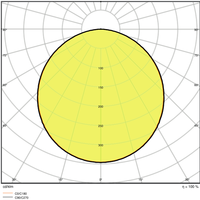
PL PFM 600 30W 4000K LDT
