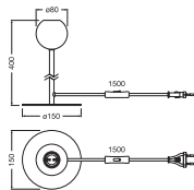
DECOR BUBBLE TABLE E27
